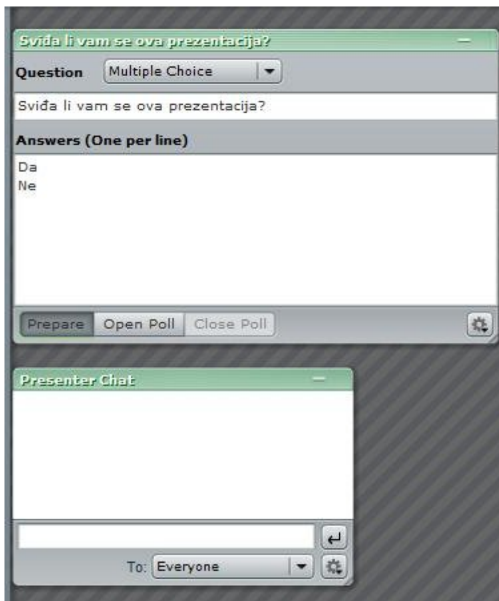
Slika 5. Priprema ankete
