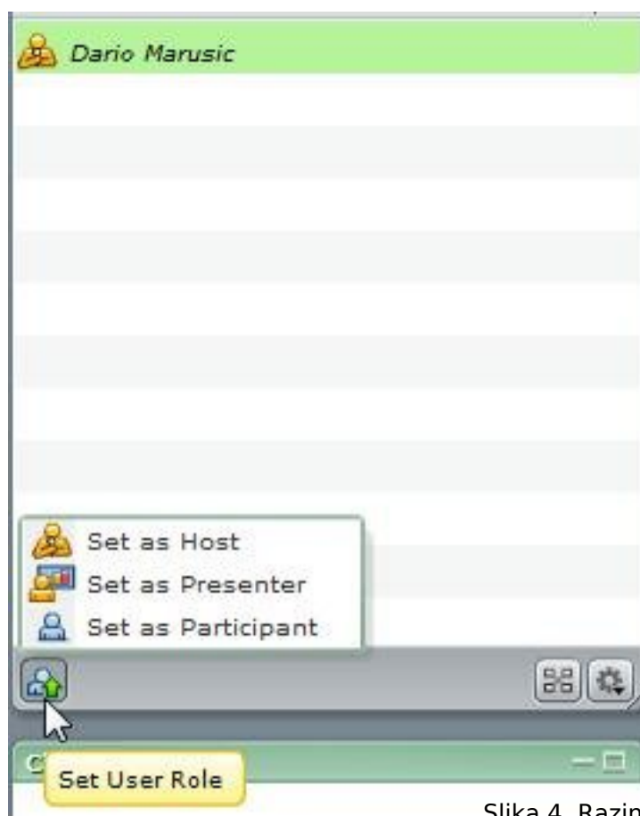
Slika 4. Razina prava
